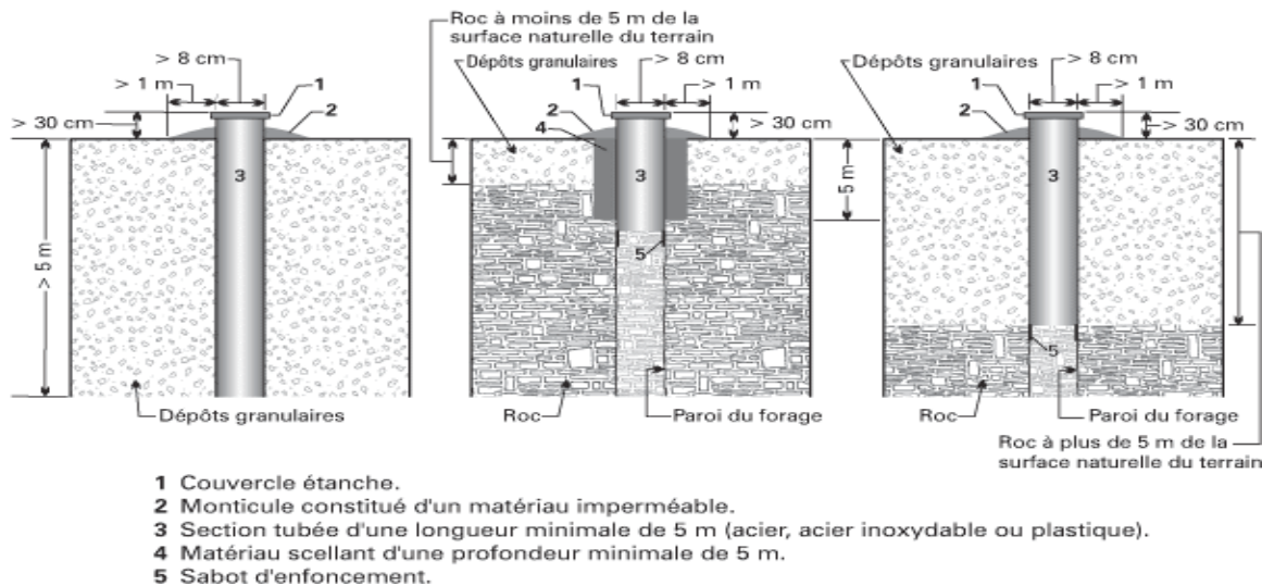
Figure 1 – Puits tubulaire
